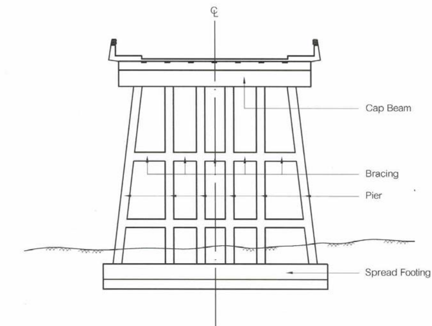
รูปที่ 1.8 Substructure และ ฐานรากของตอม่อฐานแผ่ (Spread Footing Foundation)
