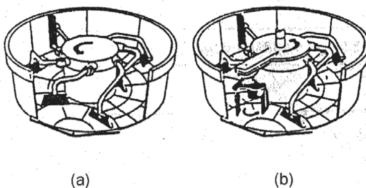
รูปที่ ค.3 Pan-Type Mixer แบบธรรมดา (a) และแบบที่มีใบกวนเพิ่ม (b)
