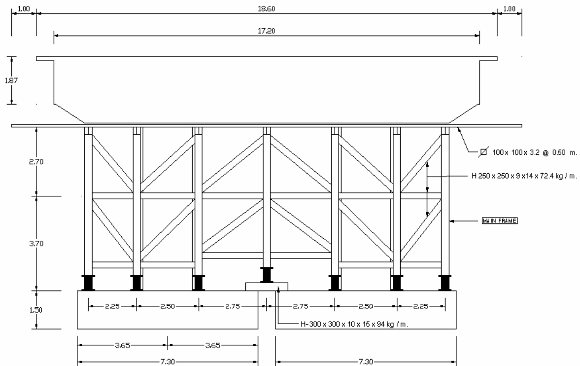
รูปที่ ข.16 (ข) การติดตั้งน้จรั้น และท้องแบบ งาน Cantilever Deck (Hollow Type)
