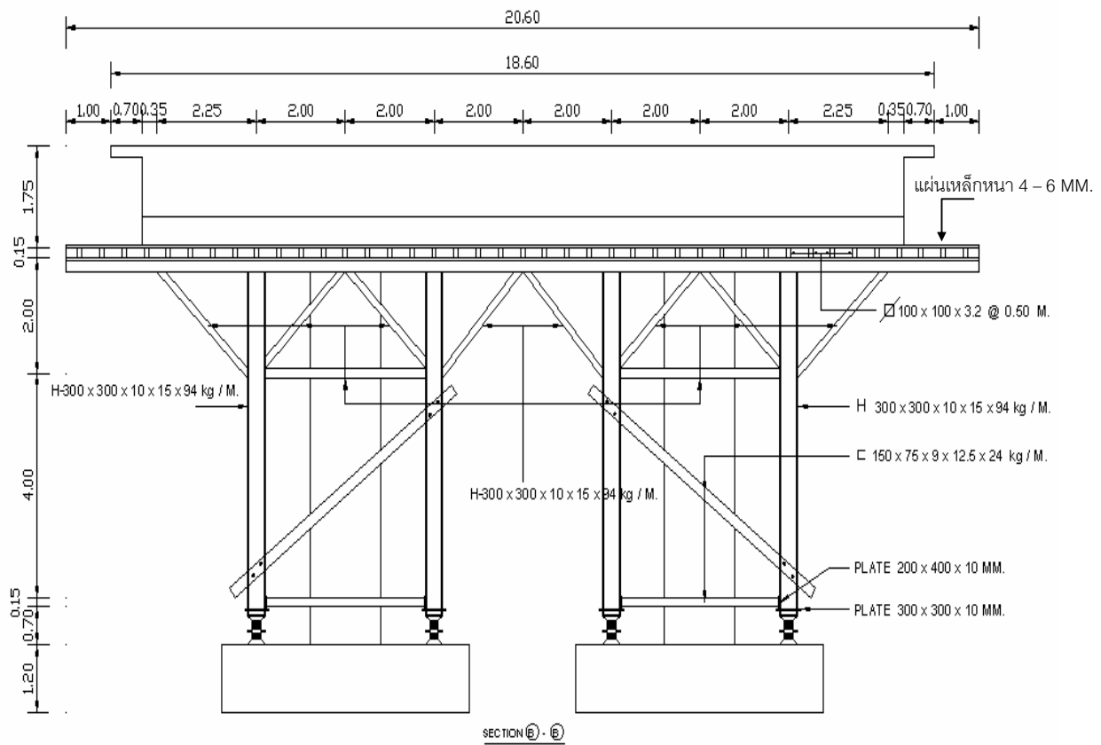
รูปที่ ข.15 (ค) การติดตั้งนั่งร้าน และท้องแบบ งาน Cantilever Deck
