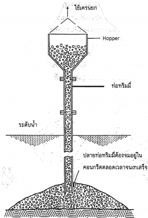
รูปที่ ก.7 การเทคอนกรีตใต้น้ำ
