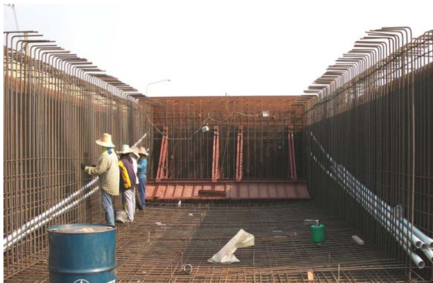
รูปที่ ข.10 ลักษณะภายในของหน้าตัดรูปกล่อง
