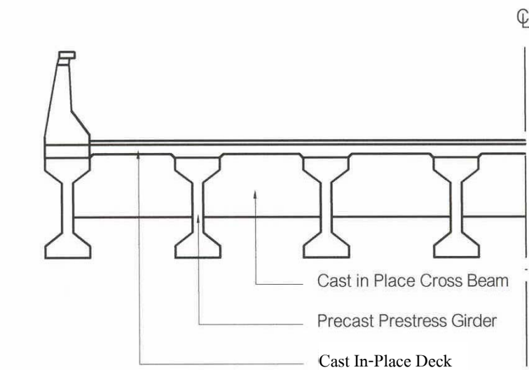
រូបភាព 1.6 Superstructure របស់ RC. Bridge Girder Type
