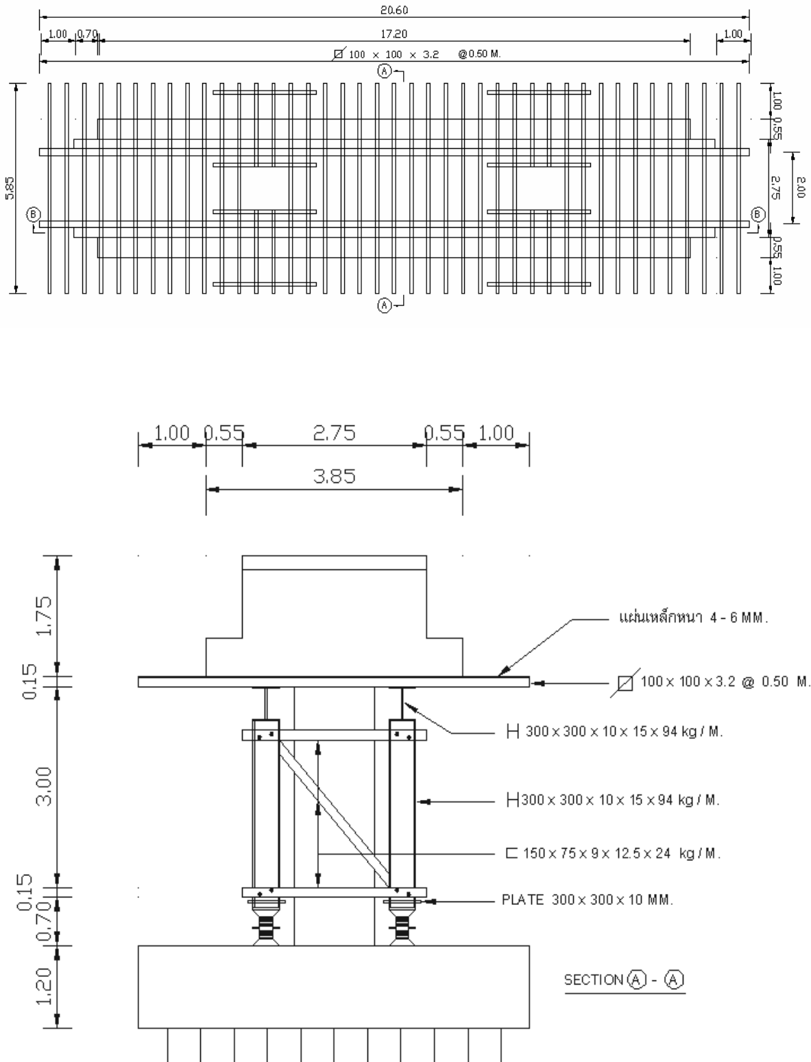
รูปที่ ข.15 (ก) การติดตั้งนั่งร้าน และท้องแบบ งาน Cantilever Deck
