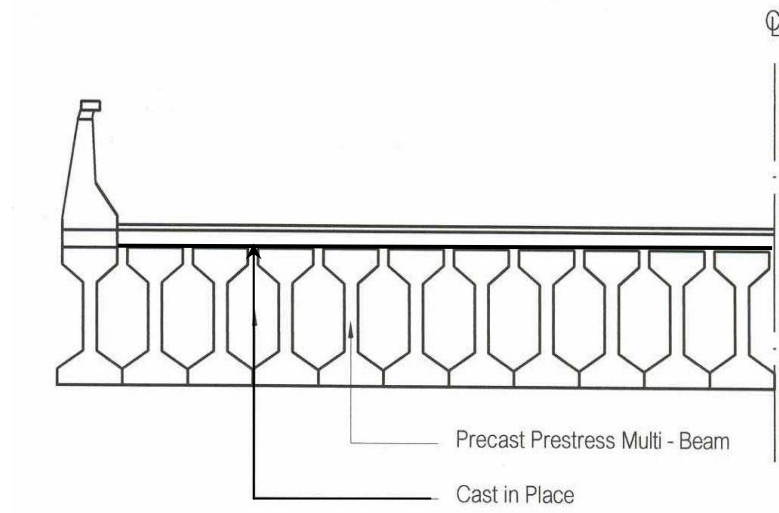
រូបភាព 1.4 Superstructure របស់ Multi - Beam Maximum Span 30.00 m.
