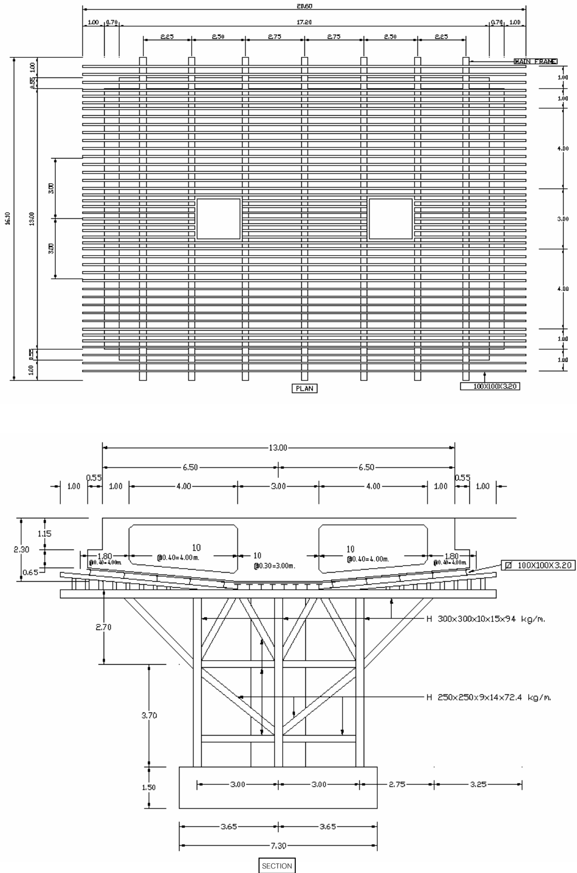
รูปที่ ข.16 (ก) การติดตั้งน้ําร้ําน และท่อดแบบ งาน Cantilever Deck (Hollow Type)
