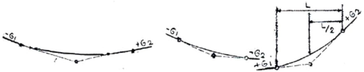
รูปที่ ก.16 โค้งทางดิ่งหงาย (Sag Vertical Curve)
