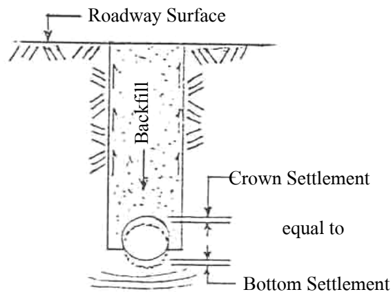
รูปที่ 11.2 กรณีวางในร่องบนฐานรากที่ทรุดตัวได้
