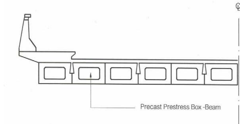
រូបភាព 1.5 Superstructure របស់ Box Beam Maximum Span 20.00 m.
