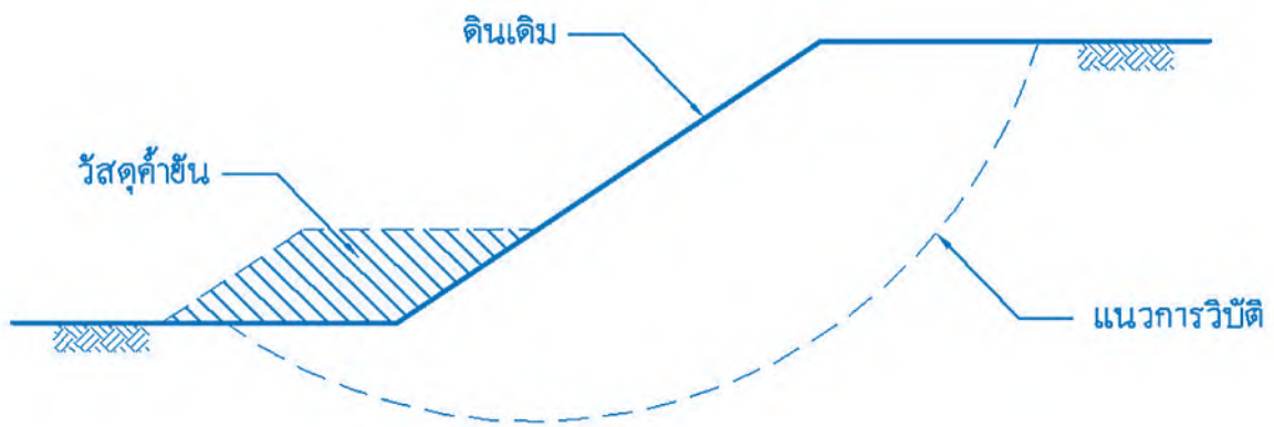
รูปที่ 2-35 การใช้น้ำหนักันบริเวณฐานพื้นที่ลาดเอียง ที่มา : มาตรฐานกรมโยธาธิการและผังเมือง (2562) 49
