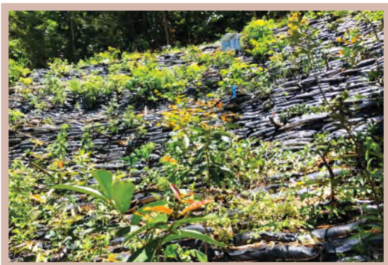
รูปที่ 3-11 การใช้กระสอบแบบมีปีกร่วมกับพืชท้องถิ่นและเสาเข็มสกรูเพื่อเสริมเสถียรภาพลาดดิน ที่มา : Jotisankasa et al. (2025) 60 บริเวณทางหลวงชนบทสาย กจ.4088 กม.16+700 อำเภอทองผาภูมิ จังหวัดกาญจนบุรี
